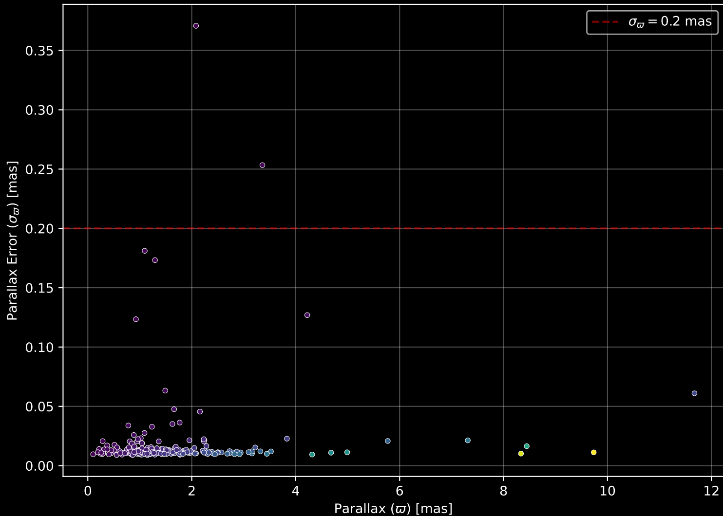
GALAH DR4 Field: [1420] Parallax Quality (n= 236)
