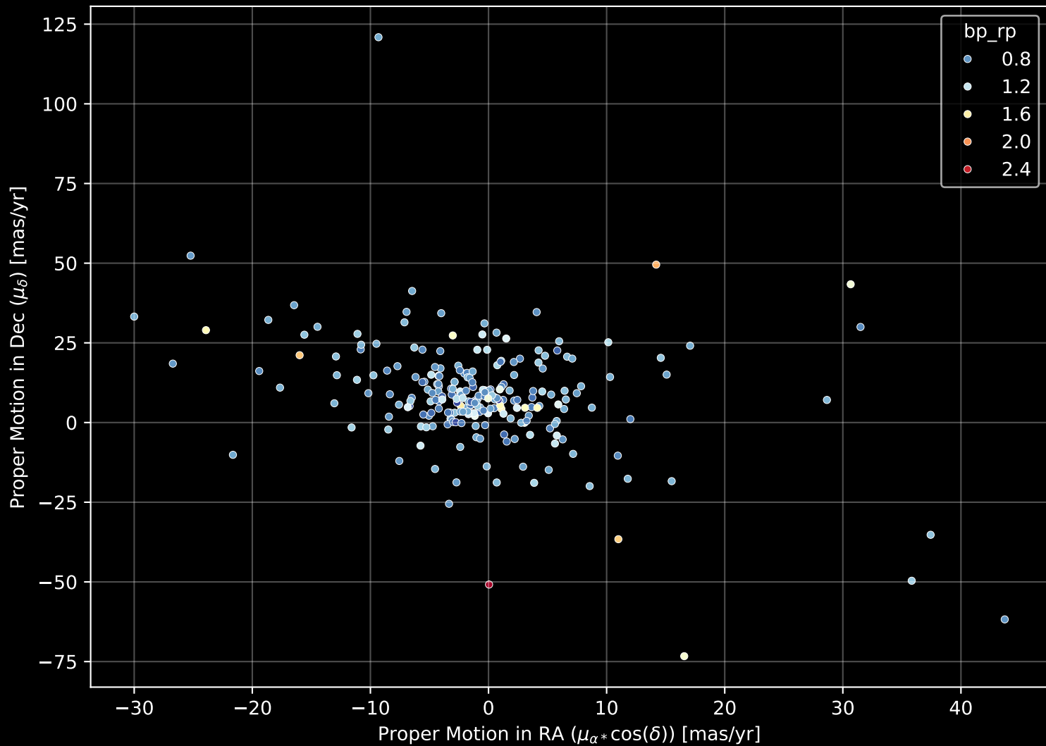
GALAH DR4 Field: [1420] Proper Motion Diagram (n= 236)
