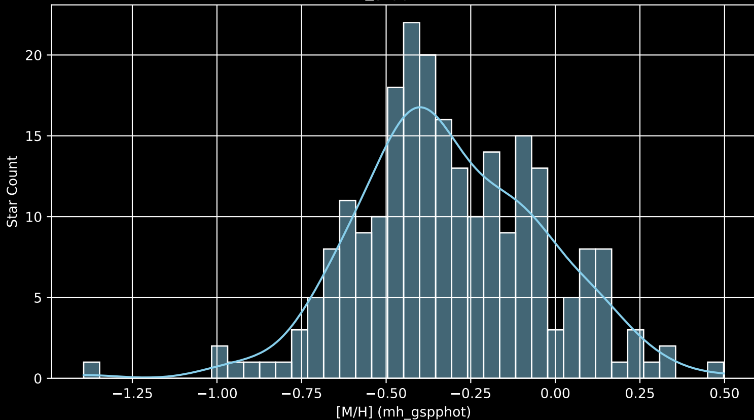
GALAH DR4 Field: [1420] [M/H] (mh_gspphot) (n= 235)
