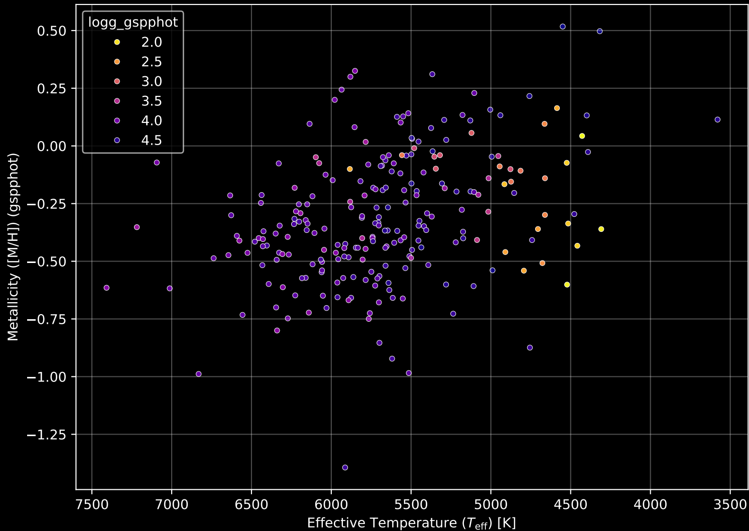
GALAH DR4 Field: [1420] Stellar Population Parameters (n= 236)
